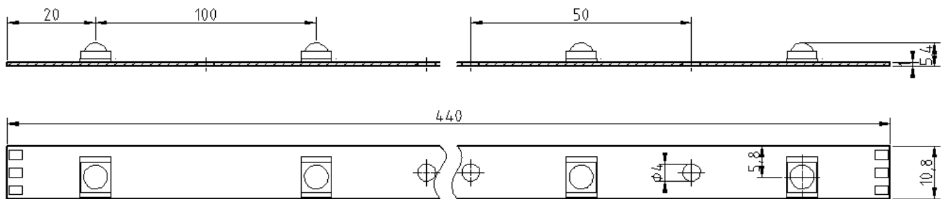
Rys. 1. Rysunek techniczny listwy LEDIS 5XR.
